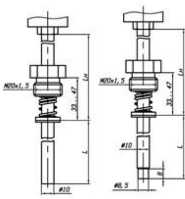
с подвижным подпружиненным штуцером («1Пр» – в записи при заказе)
