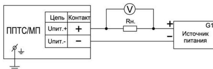
Рисунок 9.2. Схема подключения ППТС/МП к источнику питания G1, сопротивлению нагрузки R_n , вольтметру V при измерениях
