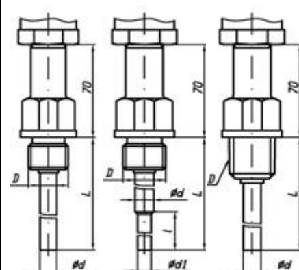
с неподвижным усиленным штуцером («2у» – в записи при заказе)
