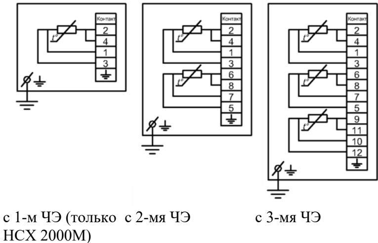
Рисунок 1.1. Схемы соединения внутренних проводов ТСМ(П) 011 с ЧЭ
