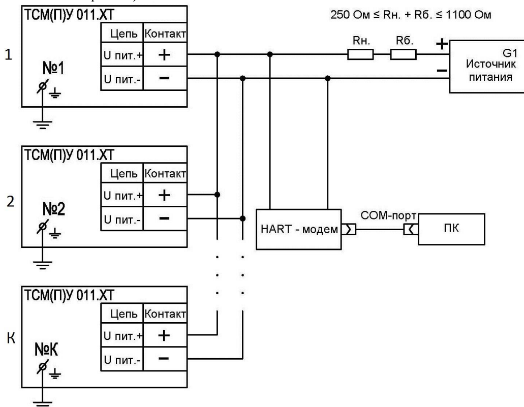
Рисунок 1.5. Схема подключений нескольких ( K \leq 15 — для ИП.ХТ с HART, версия 5, K \leq 63 - для ИП-ХТ с HART, версия 7) TCM(П)У 011-ХТ к сопротивлению нагрузки R_n , дополнительному сопротивлению R_6 , источнику питания G1, HART-модему и ПК (многооточный режим)/ Значения сопротивлений R_{мин.} и R_{макс.} для разных типов TCM(П)У 011-ХТ приведены в таблице 1.3 .
