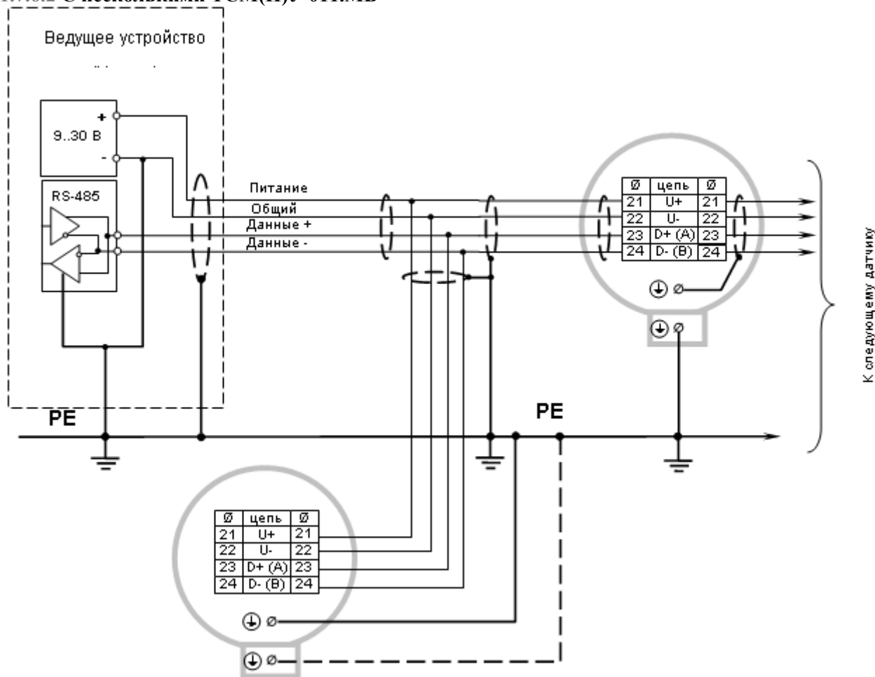
Рисунок 1.8. Схема электрических соединений при последовательном и/или параллельном подключении нескольких TSM(П)У 011.МБ
