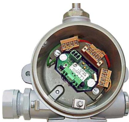
Вид на клеммную головку типа «Гб» сверху
