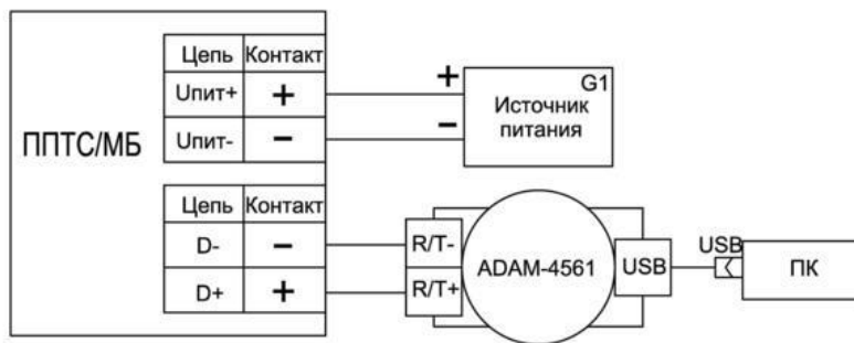
Рисунок 1.7. Схема подключения TSM(П)У.МБ к источнику питания G1, преобразователю интерфейса USB-RS-4561 и ПК при настройке и измерениях
