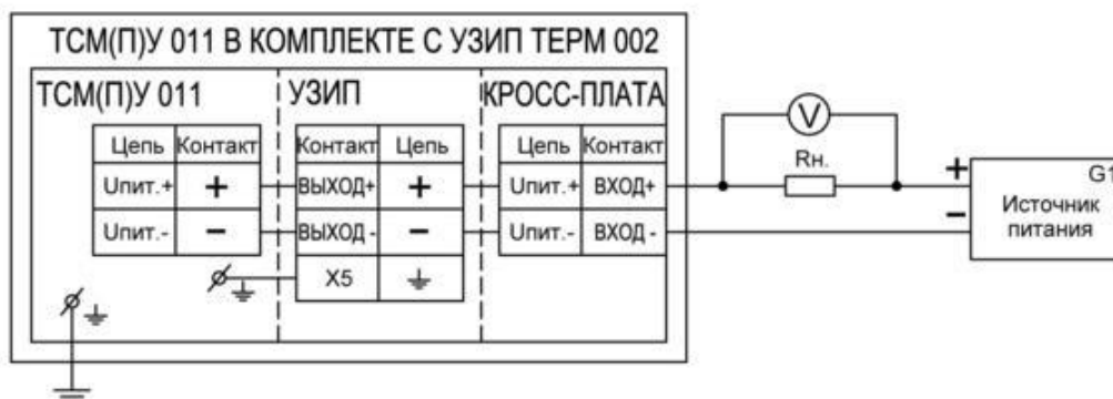
Рисунок 1.6. Схема подключений TCM(П)У 011, TCM(П)У 011.ИНД, TCM(П)У 011.МП, TCM(П)У 011.МП.ИНД, TCM(П)У 011-ХТ, TCM(П)У 011-ХТ.ИНД, TCM(П)У 011-ХТ.ИНД-СДИр с установленными в них УЗИП ТЕРМ 002
