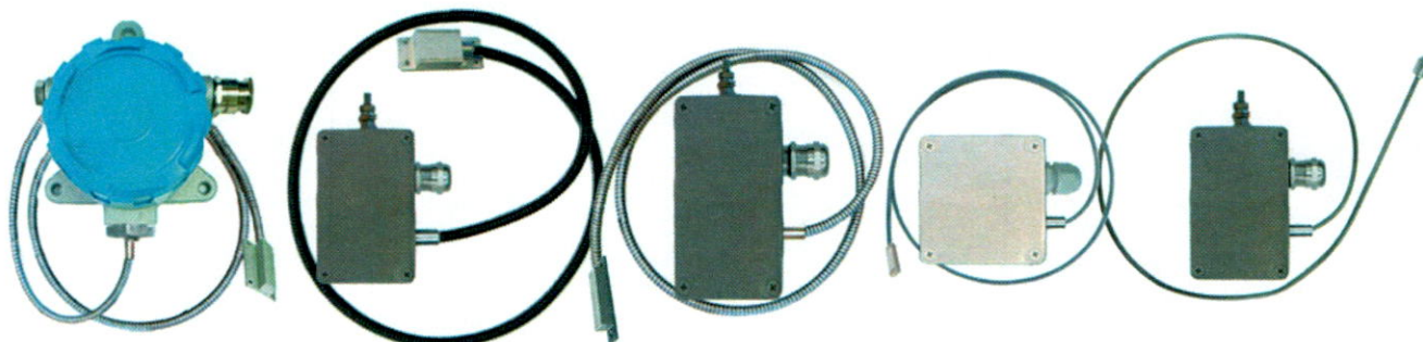
Рисунок 3 – Общий вид поверхностных общепромышленных ТС.П-Оп и взрывозащищенных ТС.П-Ex
