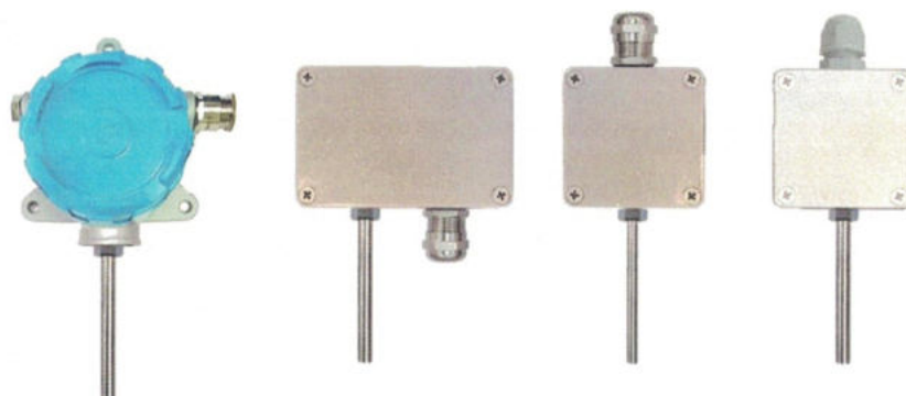
Рисунок 4 - Общепромышленные ТСп-Оп и взрывозащищенные ТСп-Ехi для измерений температуры окружающей среды (воздуха)
