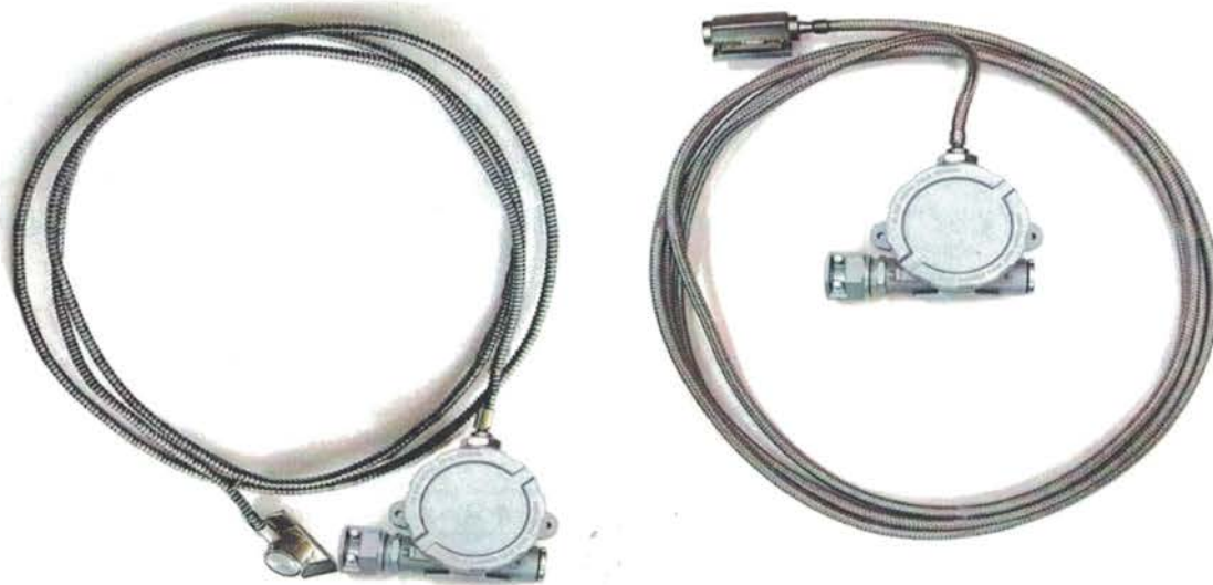
Рисунок 1 - Термопреобразователи сопротивления взрывозащищенные ТСМ 011, ТСП 011
